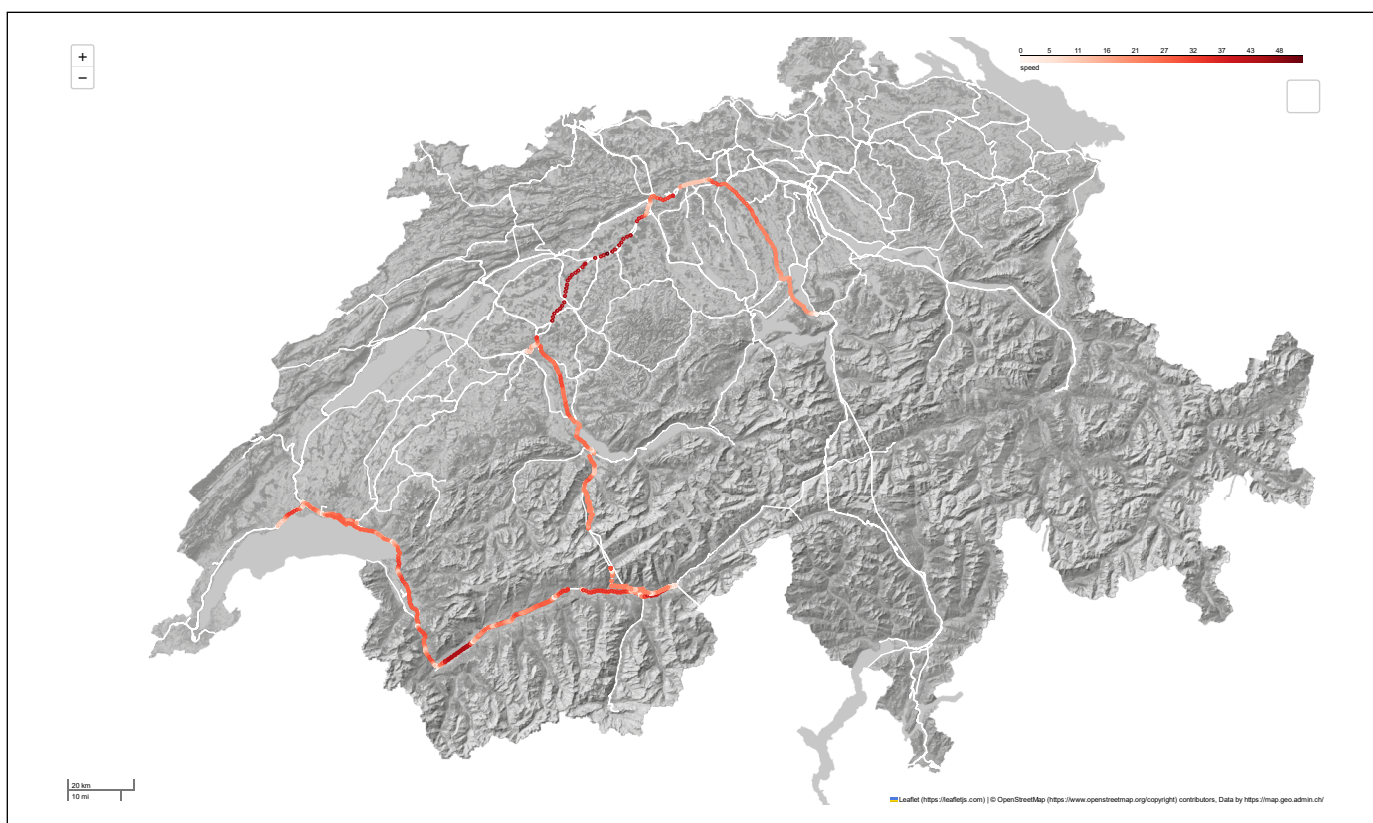
Bild 2: Messdaten einer Kampagne im November 2023 auf dem SBB-Schiennetz
