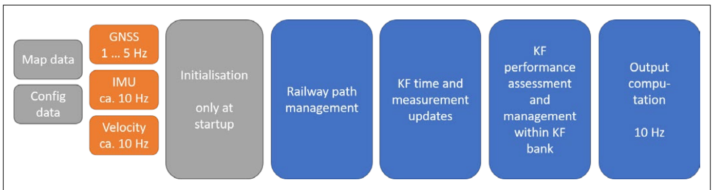
Bild 3: Struktur der KF-Bank für die Lokalisierung
